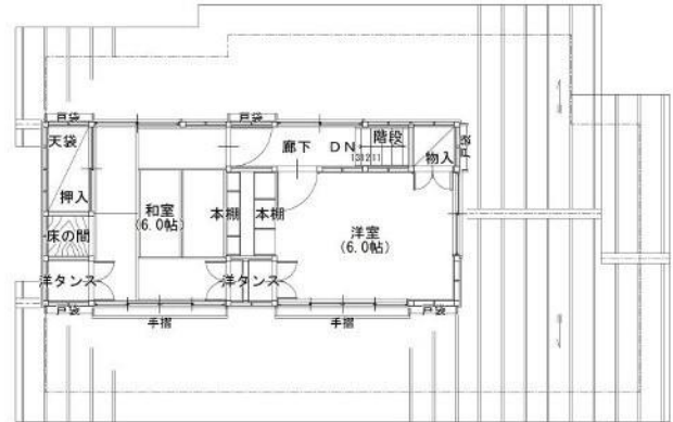
2階平面図
